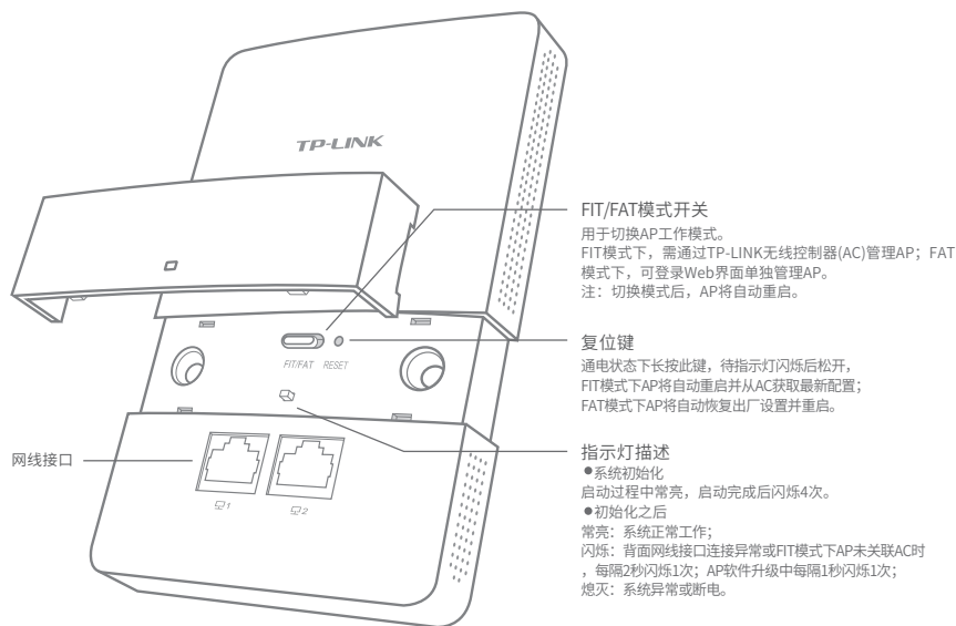
正面示意图
